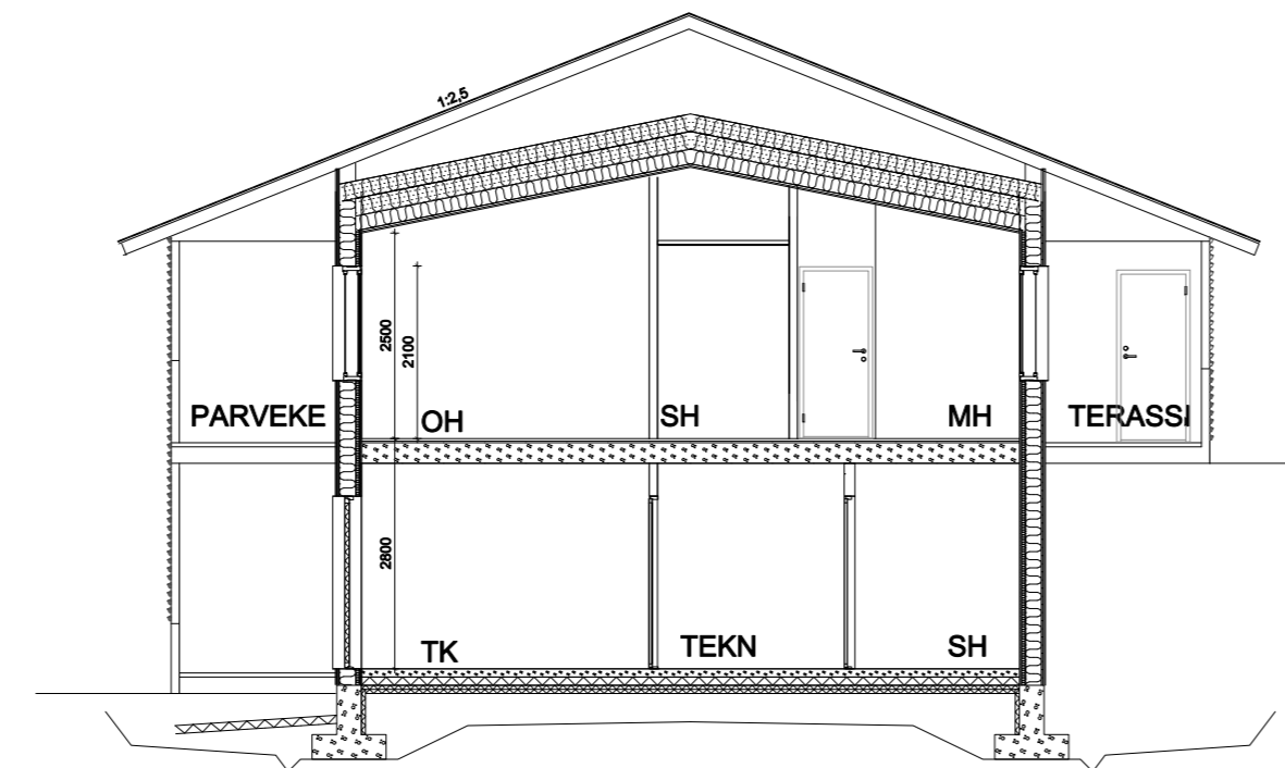
LEIKKAUS B-B
